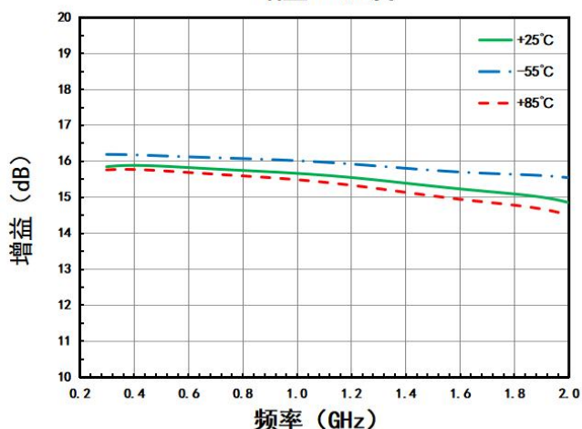
增益VS. 温度
