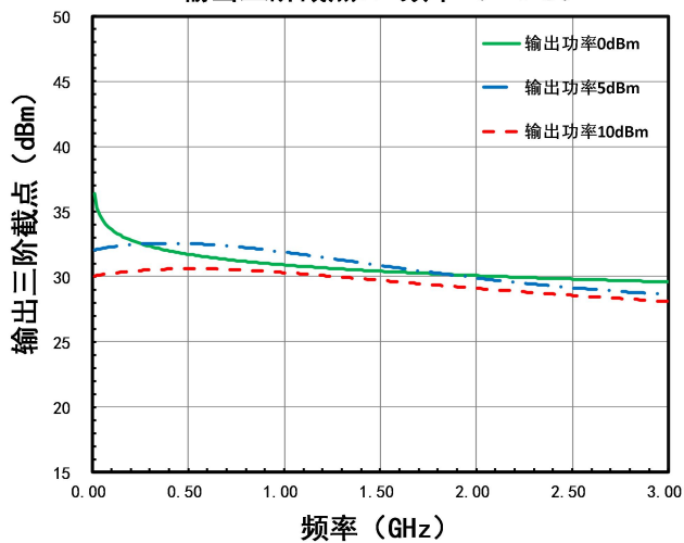
典型测试曲线: (50Ω系统, V_{dd}=+5V , I_{dd}=72mA )
