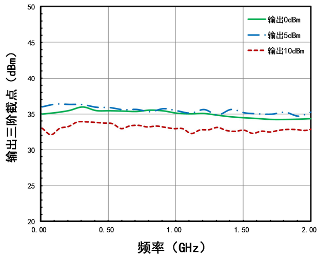
输出三阶截点VS. 频率(+25℃)
