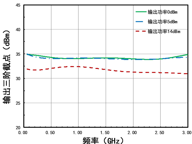
典型测试曲线 2: (50Ω系统, V_{dd}=+5V , I_{dd}=41mA , V_{G1} 接地)
