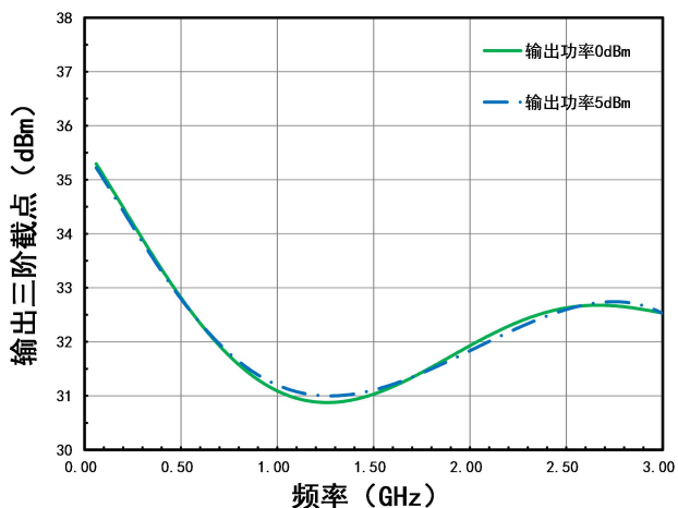
典型测试曲线: (50Ω系统, V_{dd}=+5V , I_{dd}=56mA , VG1 接地)
